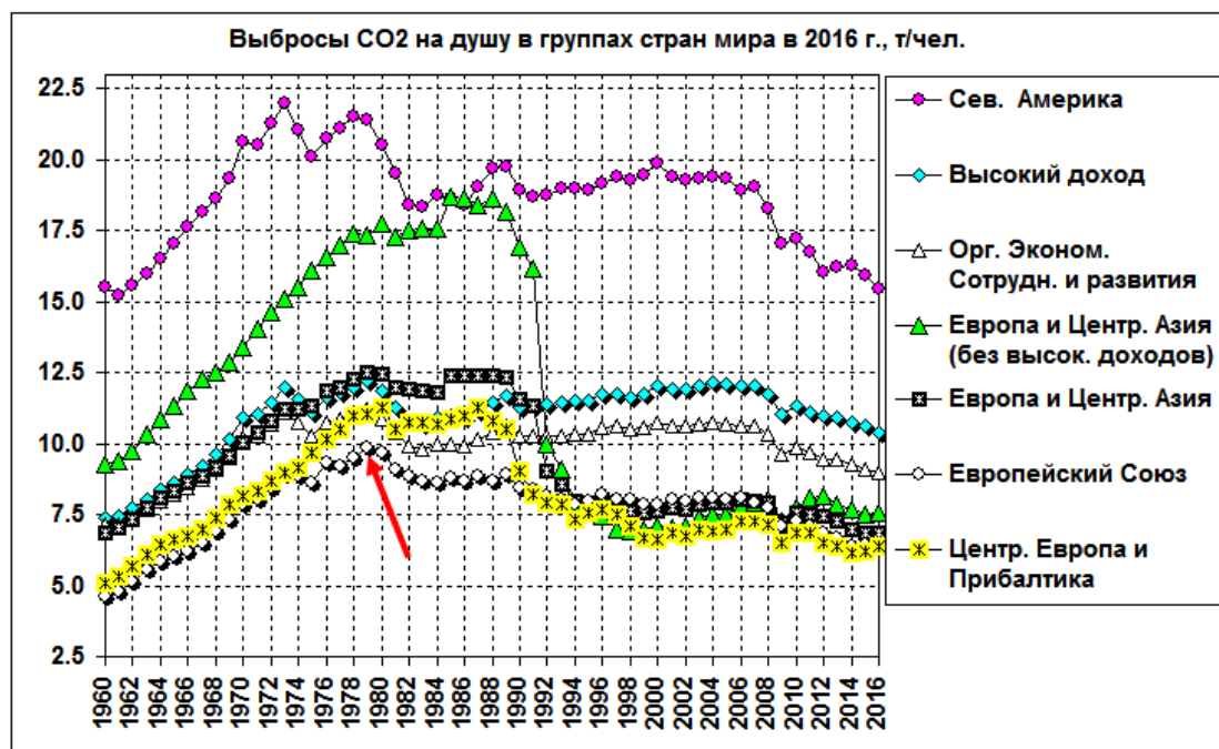
Выбросы CO 2 на душу населения нескольких групп стран мира в течение 1960-2016 гг [11]. Стрелка показывает, что минимальное значение начала спада выбросов равно 10 т С/чел. (Евросоюз)
