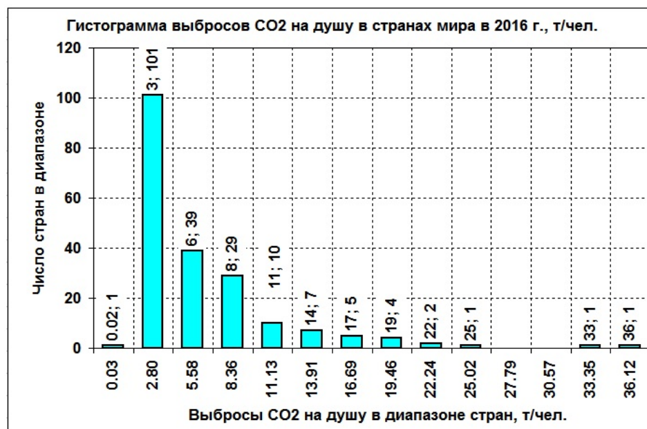
Гистограмма выбросов CO 2 на душу населения в странах мира. В подписях у столбиков указаны два значения: значение CO 2 на душу в данном диапазоне значений и число стран, попавших в него.
