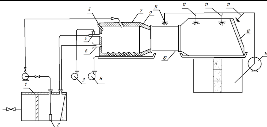
1 – гравитационный сепаратор, 2 – насос откачки жидкостной части скважинного флюида (ПРВП 63/22.5. ГОСТ 8388-72), 3 – вентилятор запальной горелки (ВВД-5), 4 – запальная горелка (ГНП-7), 5 – электрозапальник, 6 – основная (инжекционная) горелка, 7 – топочное устройство, 8 – вентилятор дутьевой (ВДН-8), 9 – переходное кольцо к оросительному теплообменнику, 10 – оросительный теплообменник, 11 – эвольвентные оросители (ЭО-16-25), 12 – сетчатый брызгоотделитель, 13 – основной водовод
