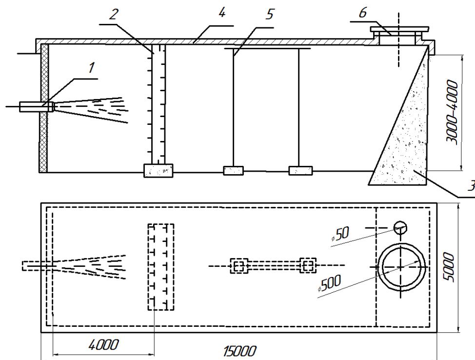
1 – факельный отвод, 2 – турбуляризирующие решетки, 3 – отбойная бетонная плита, 4 – герметизирующее покрытие, 5 – опоры покрытия, 6 – фланец выхода газа в топку
