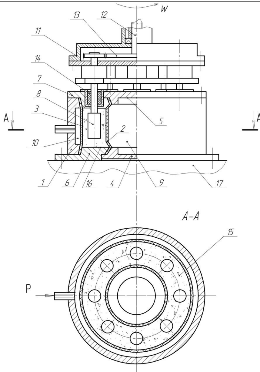
Рисунок 1- Схема устройства для обработки сложнопрофильных деталей из порошковых материалов.
